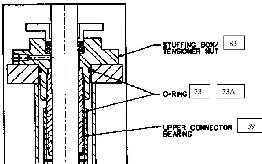
Afbeelding 7-E MONTAGE SPANNERMOER
